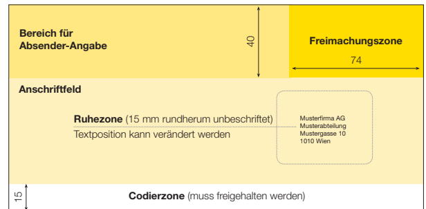
Muster für Sendung im Format C6/5
